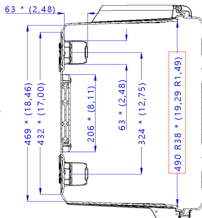
Sezione B-B Sezione B-B
