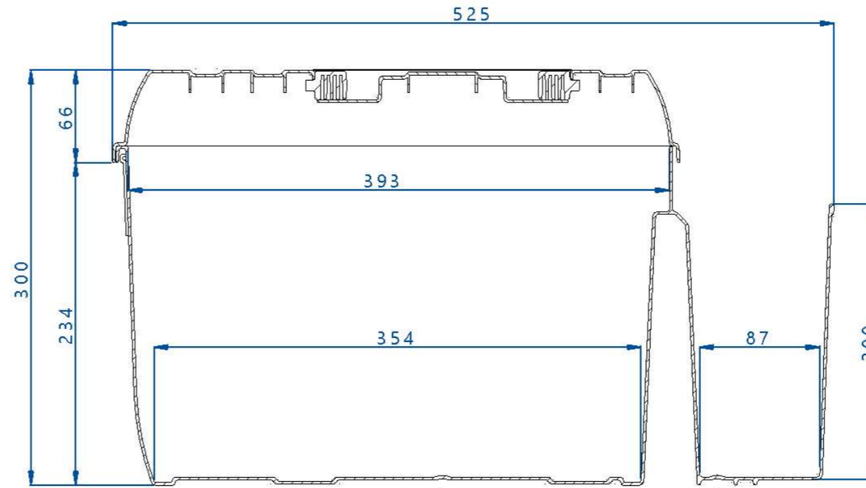
SEZIONE A-A
