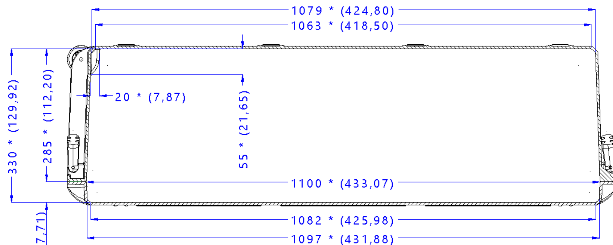
Sezione A-A
