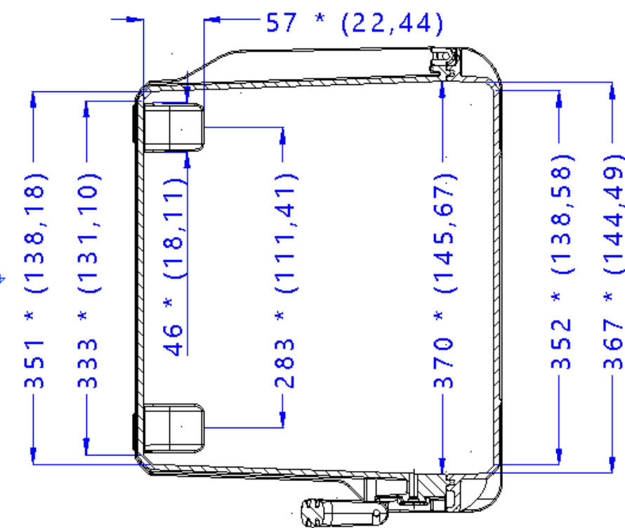
Sezione B-B
