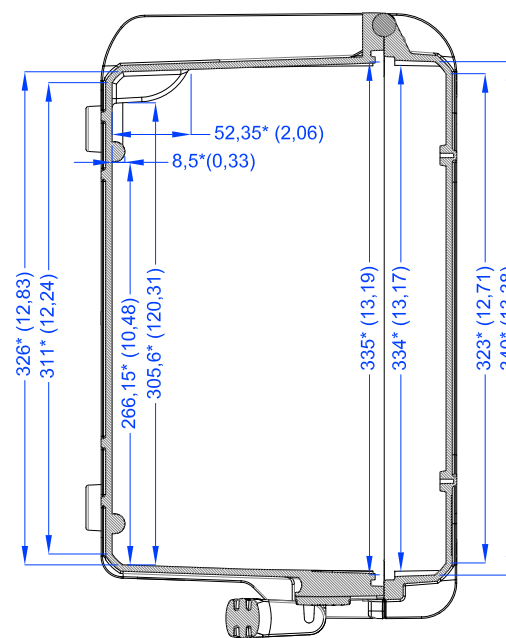
Sezione B-B Section B-B
