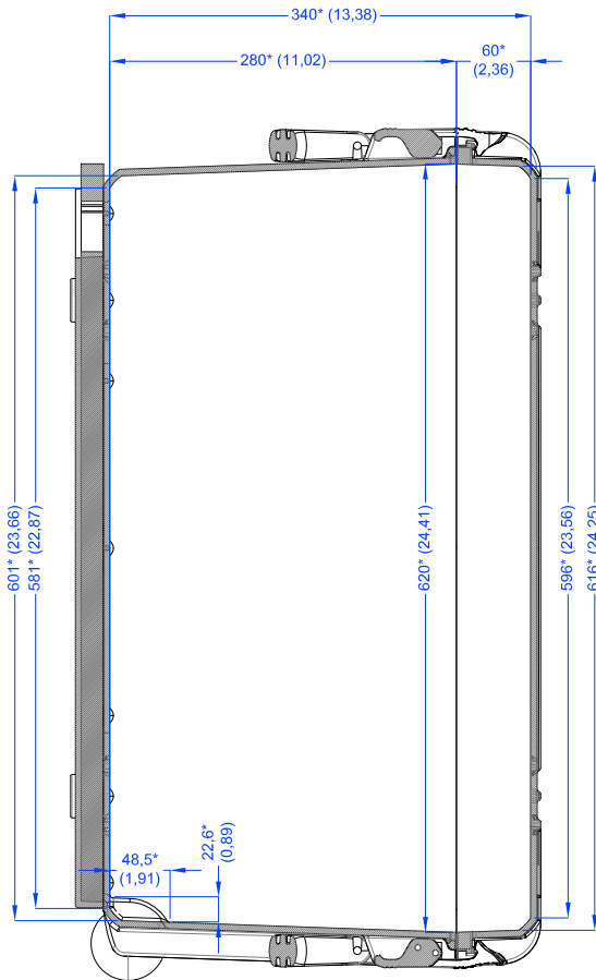
Sezione A-A
