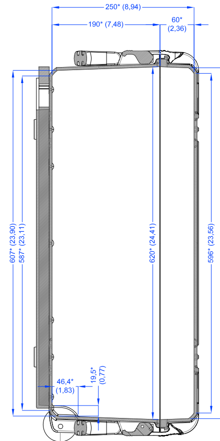
Sezione A-A Section A-A
