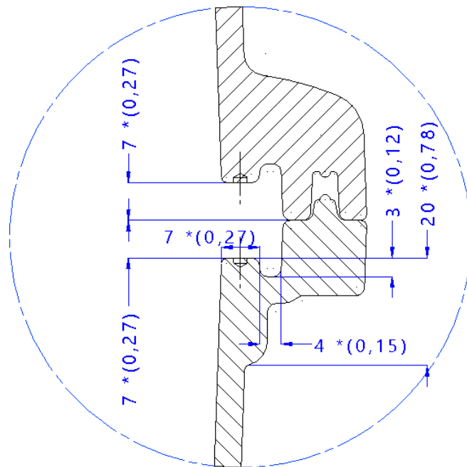
Dettaglio chiusura ermetica Lid Airtight Closure Detail
