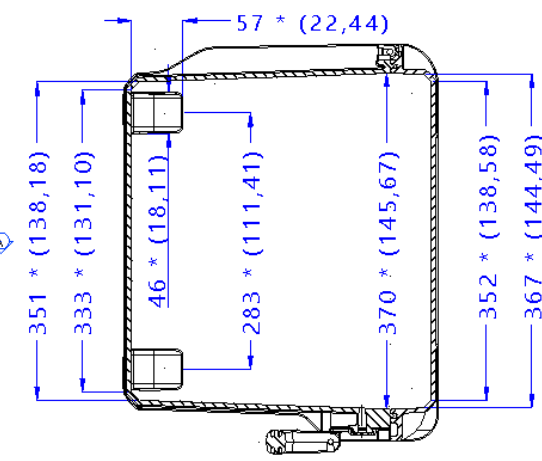
Sezione B-B Section B-B
