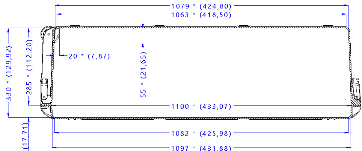
Sezione A-A Section A-A
