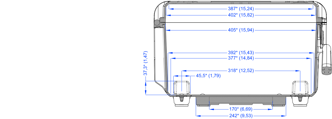
Sezione B-B
