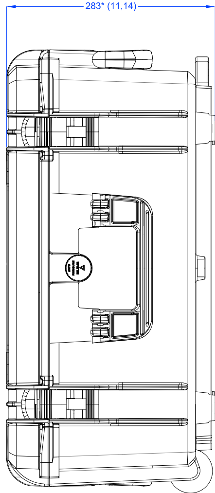
Lato Apertura Opening Side
