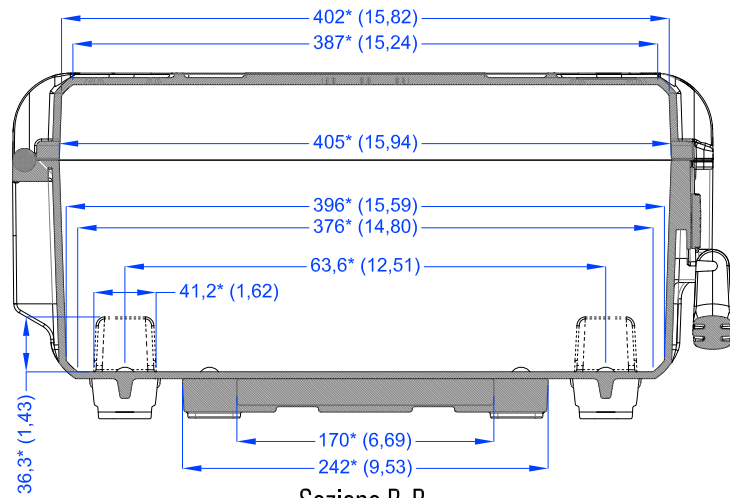
Sezione B-B Section B-B
