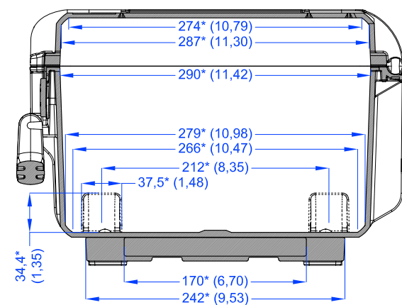
Sezione B-B Section B-B
