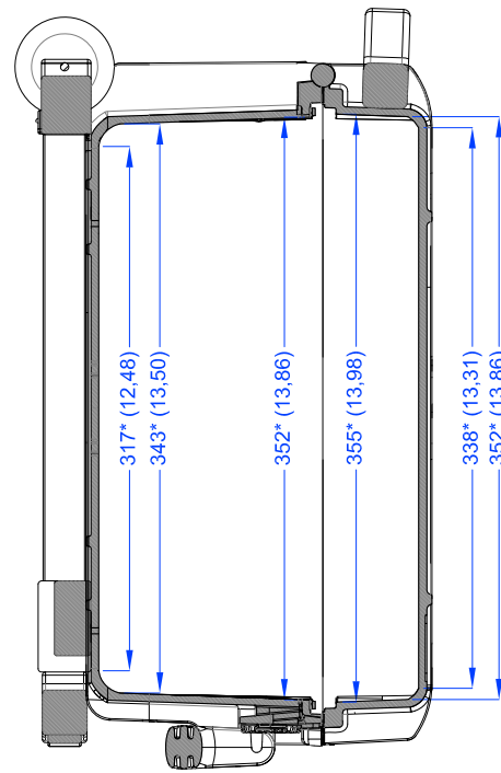
Sezione B-B Section B-B
